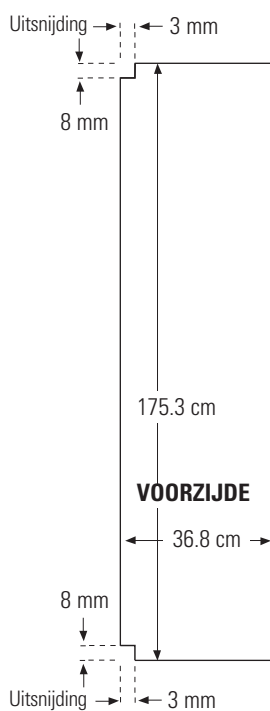
Paneel van vriesvak zonder verdeler
