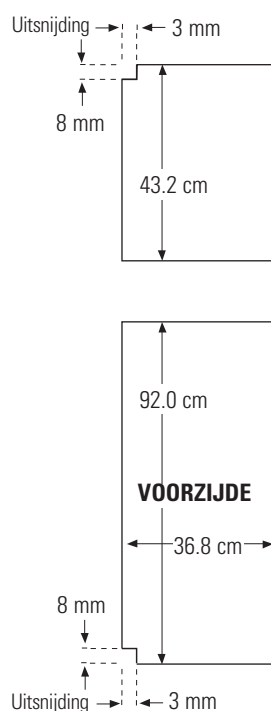
Paneel van vriesvak met verdeler
